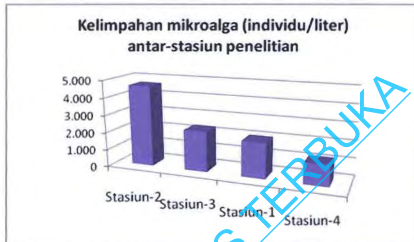
Gambar 4. Histogram indeks kelimpahan spesies mikroalga antar-stasiun penelitian
