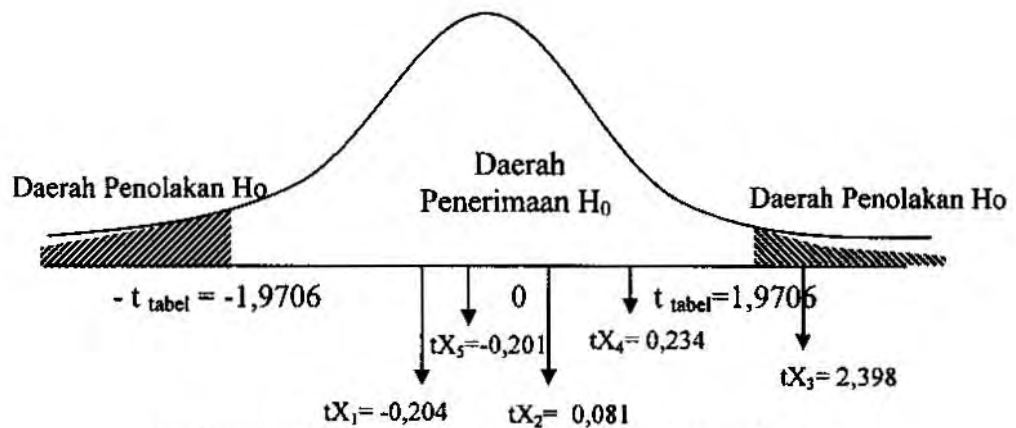
Gambar 4. Daerah penerimaan dan penolakan H_0 uji t
