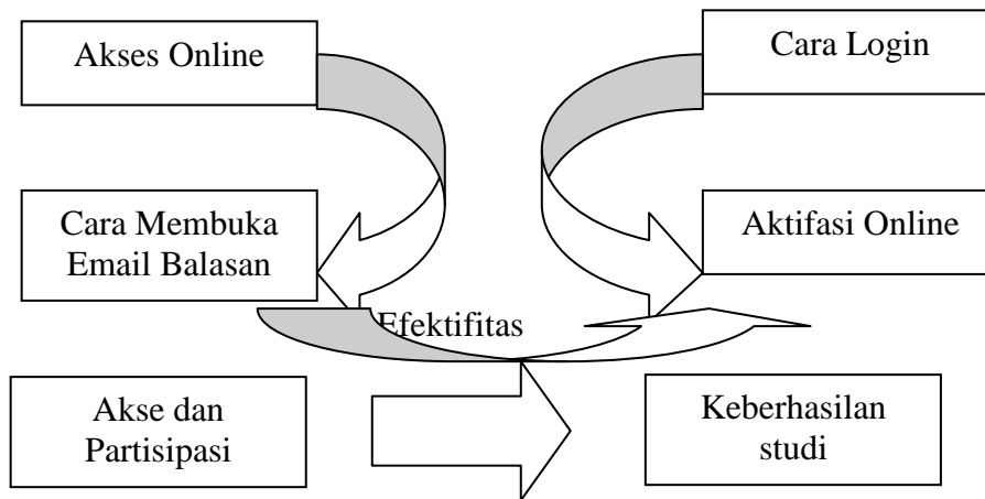
Gambar 3.1. Kerangka Pemikiran
