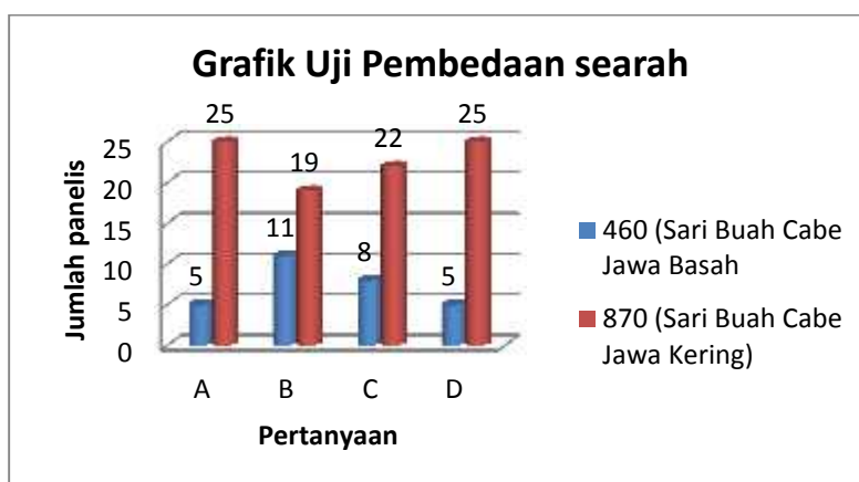
Gambar 3. Grafik uji pembedaan searah antara sari buah cabe jawa basah dan sari buah cabe jawa kering.
